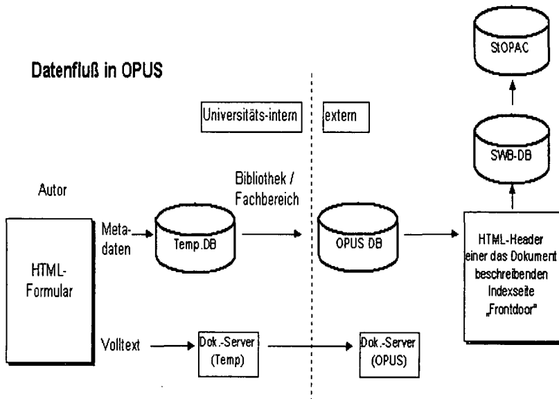
Abb. 3: Datenfluß im Online Publikationsverbund der Universität Stuttgart
